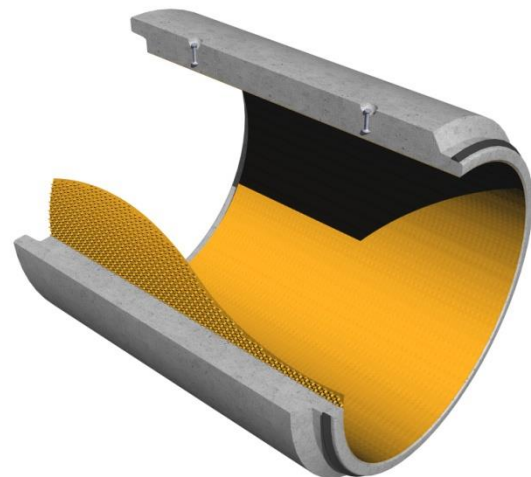
Tubo prefabbricato giunto a spessore con rivestimento in PE 'liner'
