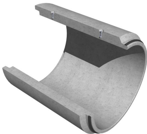
Tubo prefabbricato giunto a spessore
